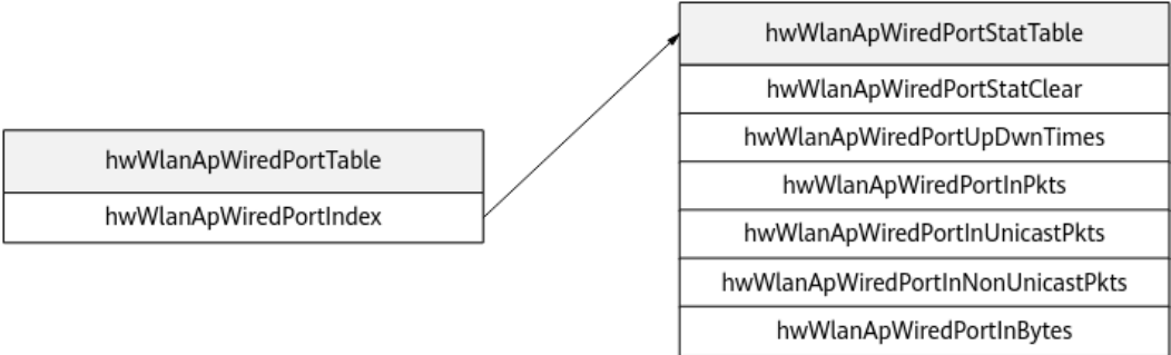
图 138-2 hwWlanApWiredPortTable 和 hwWlanApWiredPortStatTable 的表间关系
