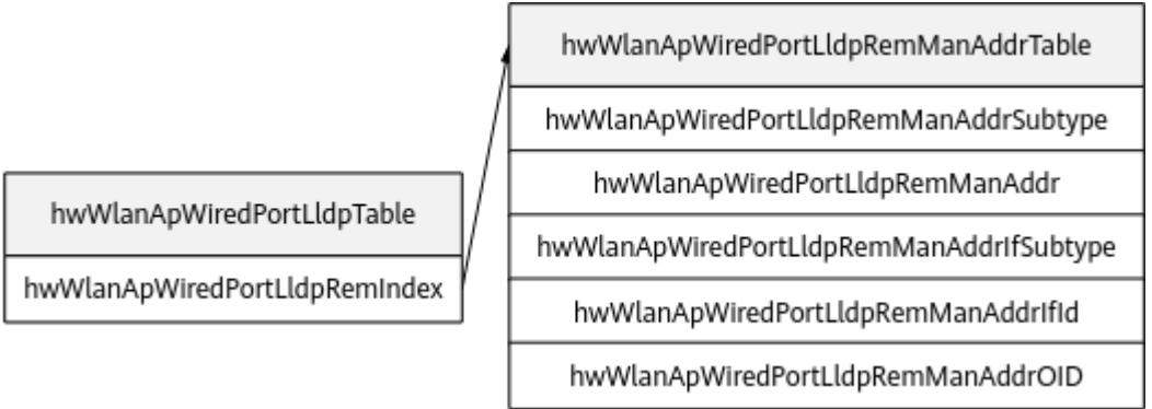
图 138-3 hwWlanApWiredPortLldpTable 和 hwWlanApWiredPortLldpRemManAddrTable 的表间关系
